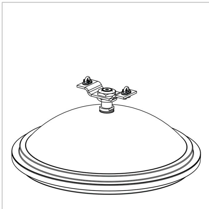
CITEA GEN3 | Montagem suspensa ajustável 1" gás macho (S4)
